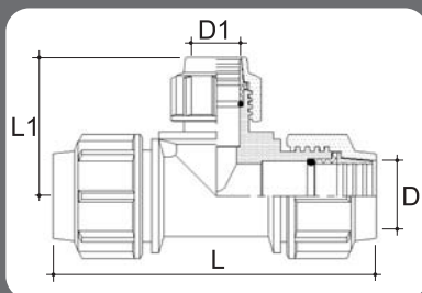
REDUCING TEE (R.T.) 大小梯
