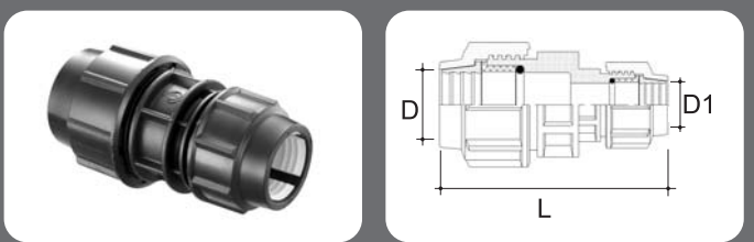
REDUCING COUPLER (R.C) 大小梳吉
