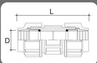
STRAIGHT COUPLER (S.C) 梳吉
